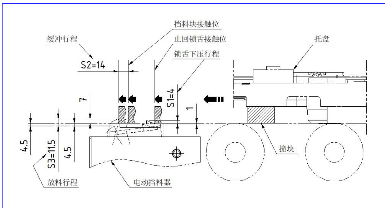
图 3-- 运动关系尺寸图
