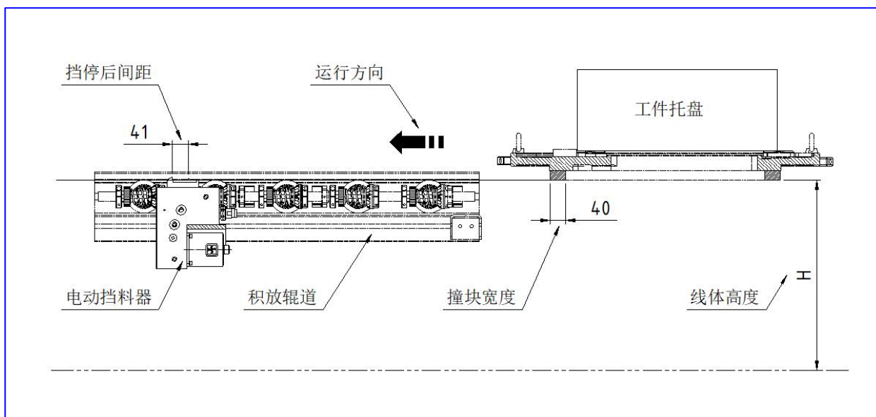
图 2-- DLXD-PT700-40 电动挡料器与托盘撞块尺寸关系图
