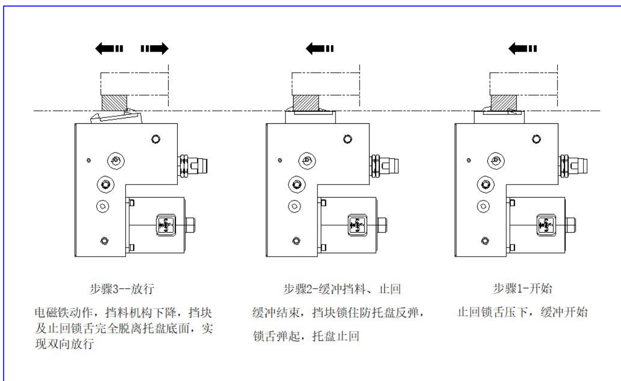
图 4-- 动作过程分解图
