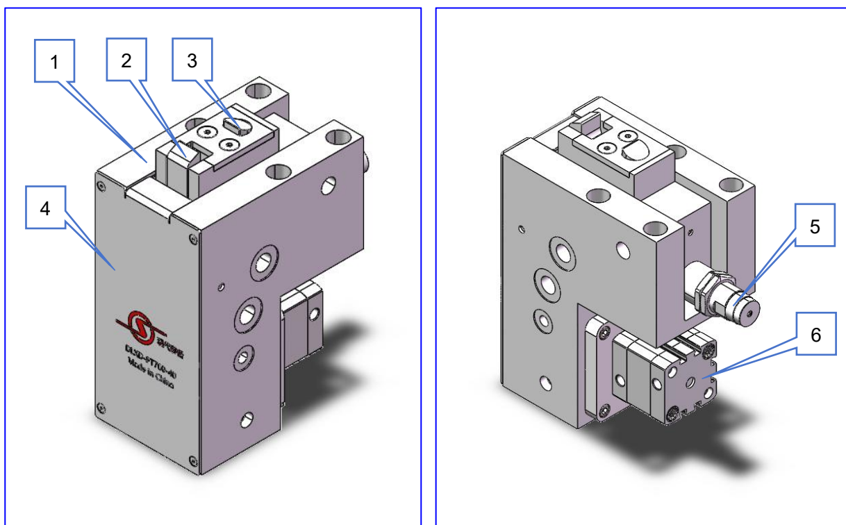
图 1-- DLXD-PT700-40A 气动挡料器构成图
