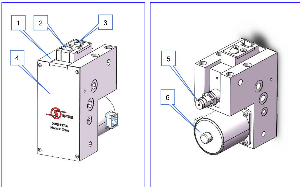
图 1-- DLXD-PT700-40E 电动挡料器构成图
