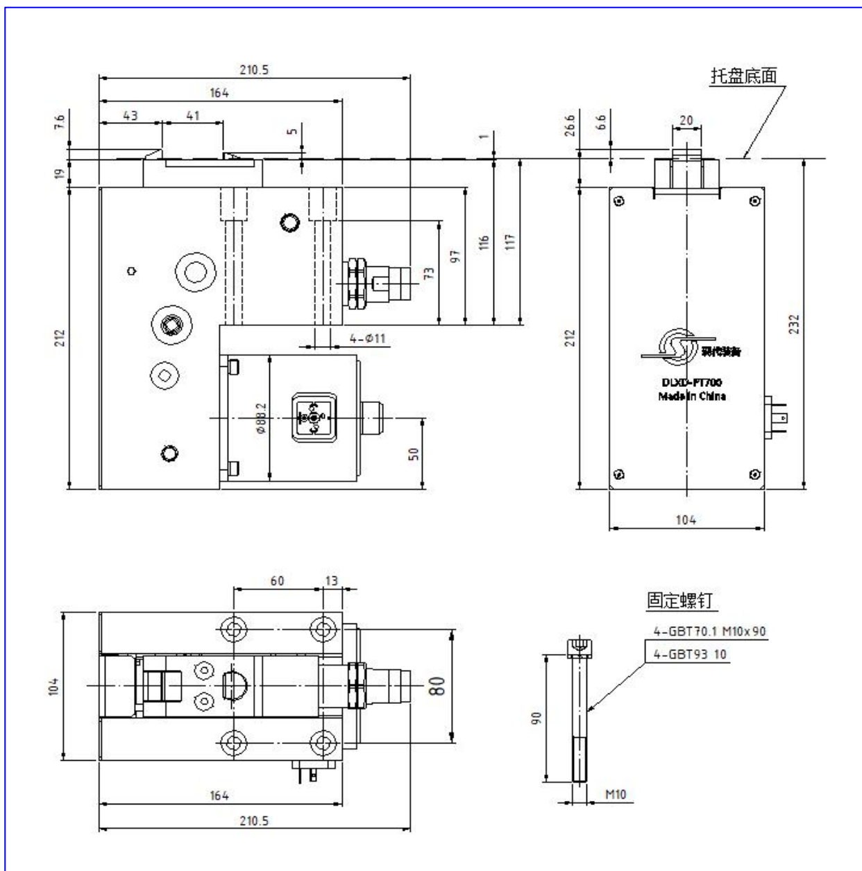
图 5- DLXD-PT700-40E 安装尺寸图
